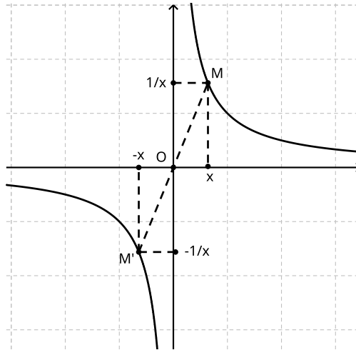
Figure 1: L'hyperbole d'équation y = 1/x
